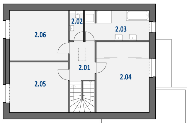
PŮDORYS 2.NP
