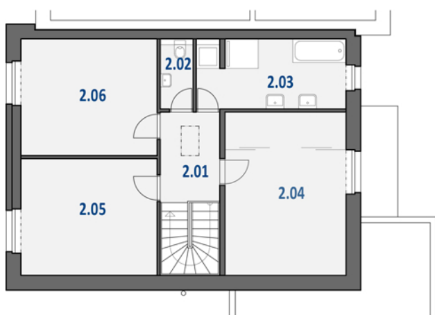
PŮDORYS 2.NP
