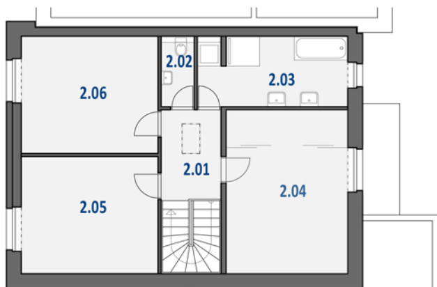
PŮDORYS 2.NP
